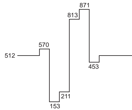
NTSC, Setup
