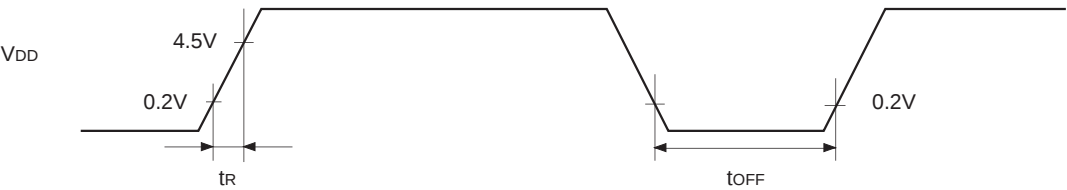
Fig. 9. Power-on reset
