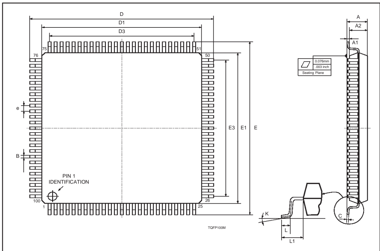
TQFP100
